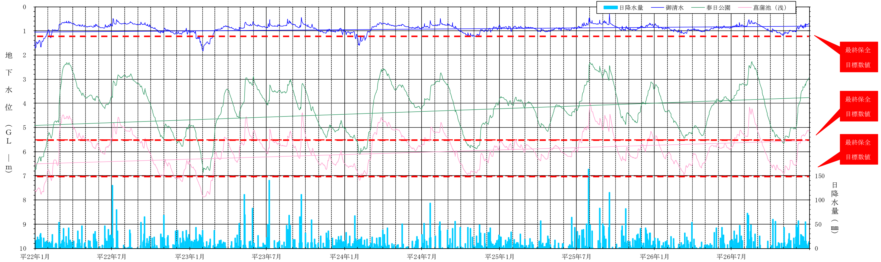
[ 3 観測井の地下水位変動グラフ (平成 22 年～26 年 5 年間) ]
