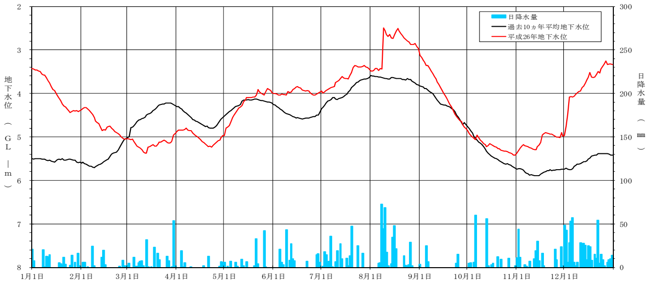
[ 平成 26 年地下水位変動グラフ 幸町観測井 (NO. 10) ]
