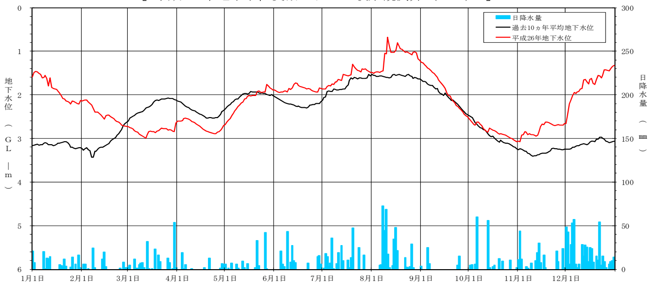
[ 平成 26 年地下水位変動グラフ 駅東観測井 (NO. 5) ]
