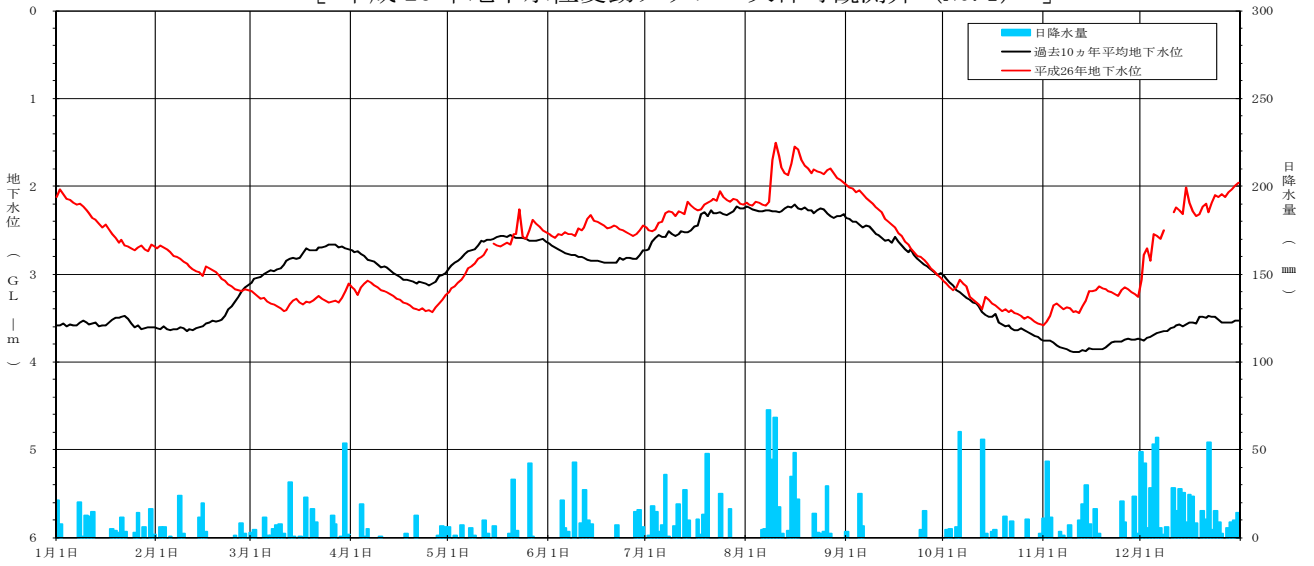
[ 平成 26 年地下水位変動グラフ 天神町観測井 (NO. 1) ]
