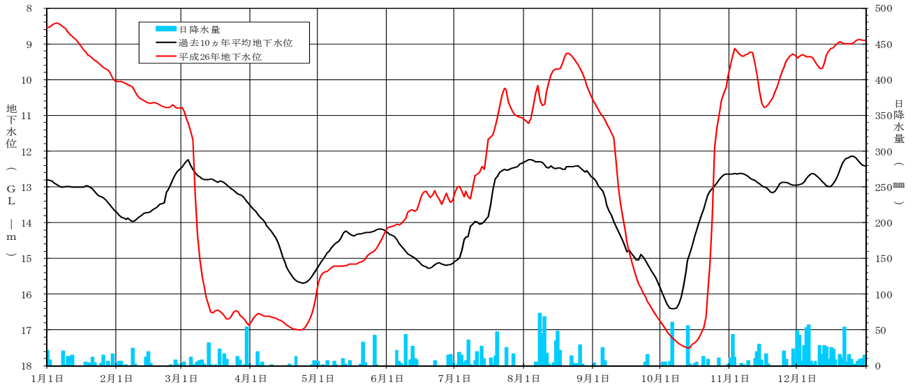
[ 平成 26 年地下水位変動グラフ 木本原下観測井 (NO. 28) ]
