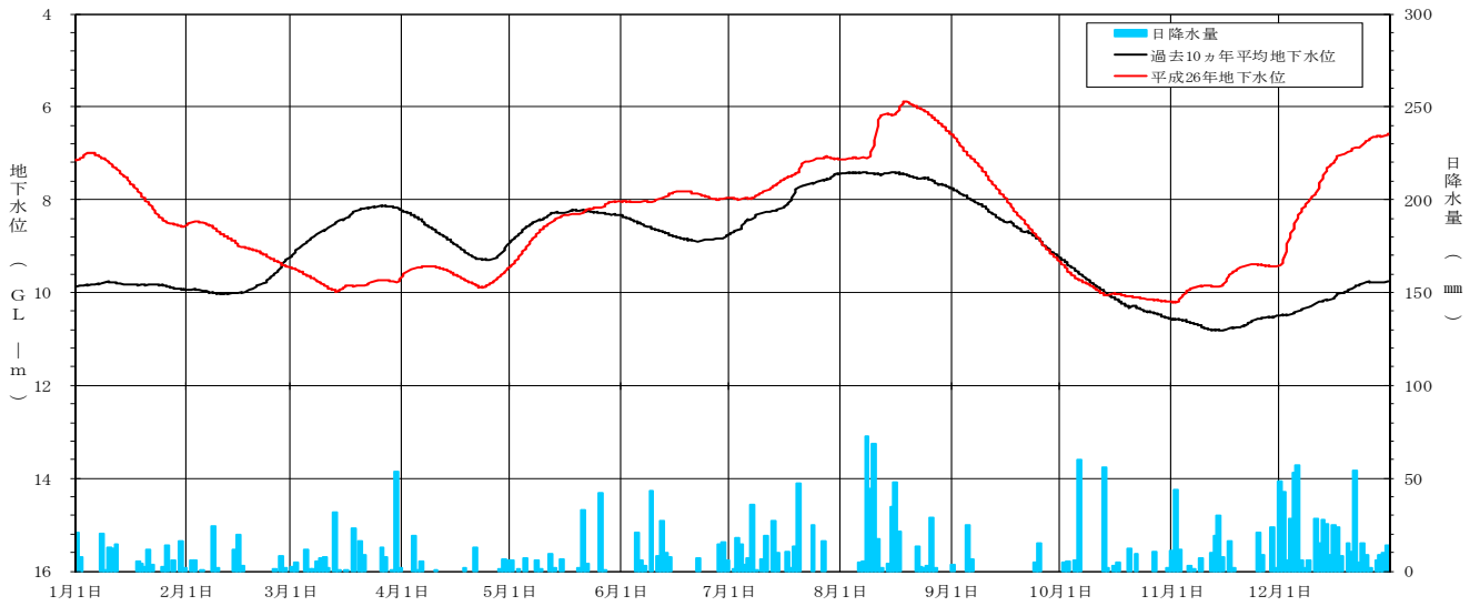
[ 平成 26 年地下水位変動グラフ 篠座観測井 (NO. 16) ]
