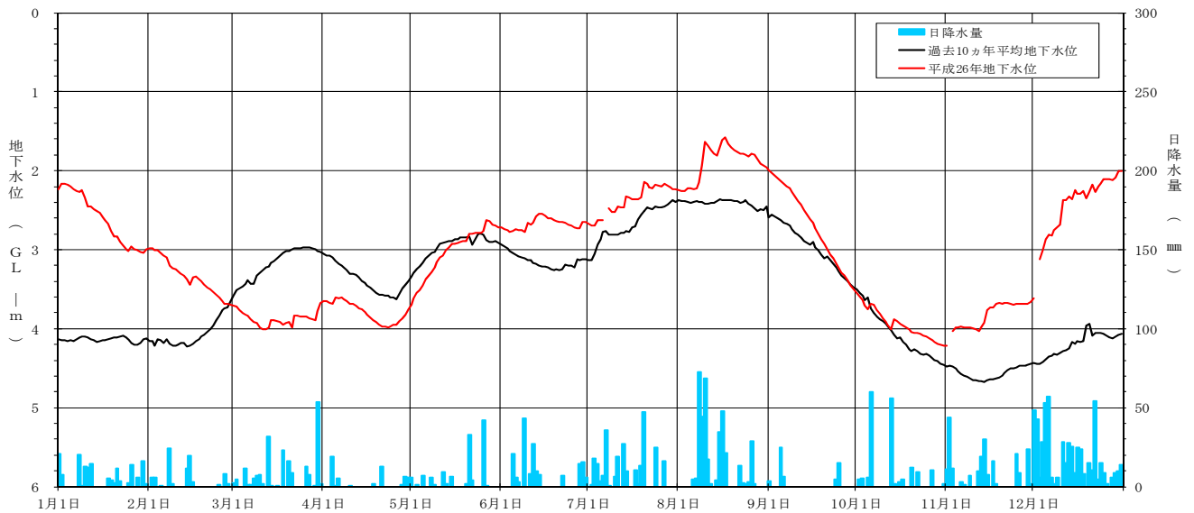
[ 平成 26 年地下水位変動グラフ 本願清水観測井 (NO. 13) ]
