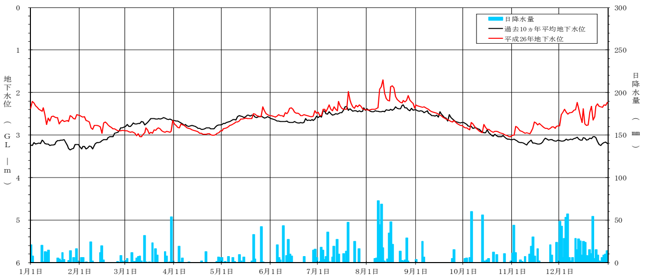
[ 平成 26 年地下水位変動グラフ 石灯笼観測井 (NO. 12) ]
