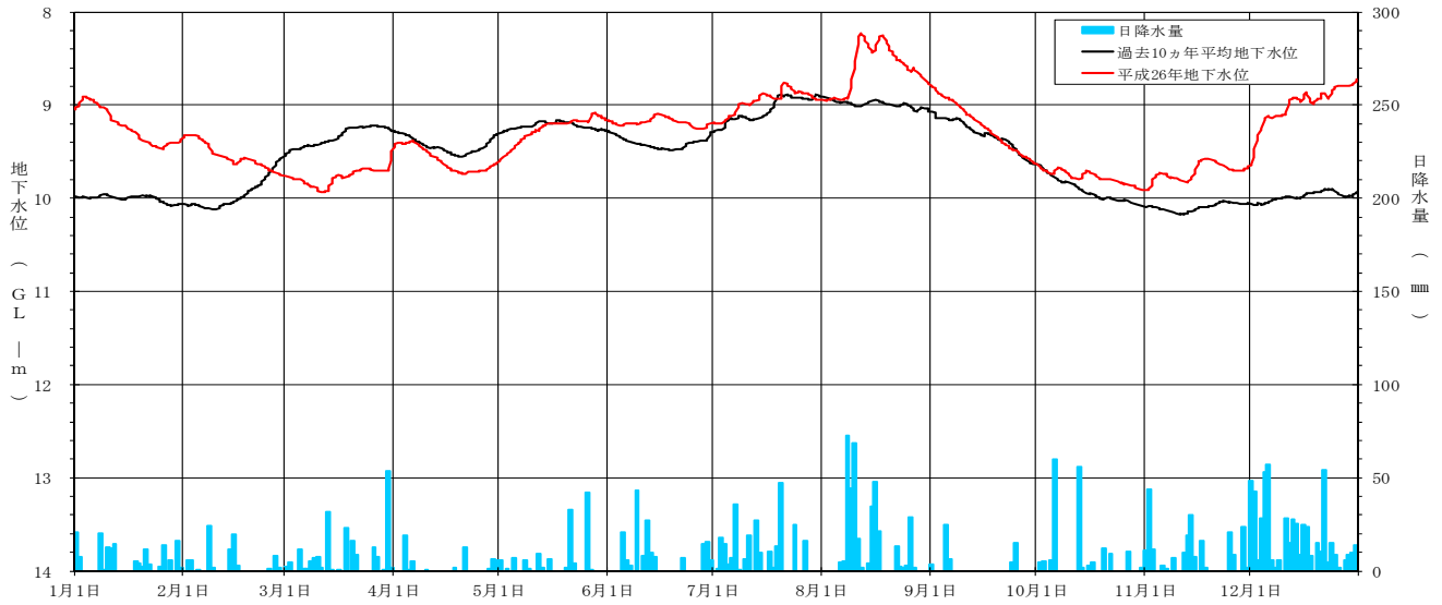
[ 平成 26 年地下水位変動グラフ 菖蒲池（深）観測井（NO. 22） ]
