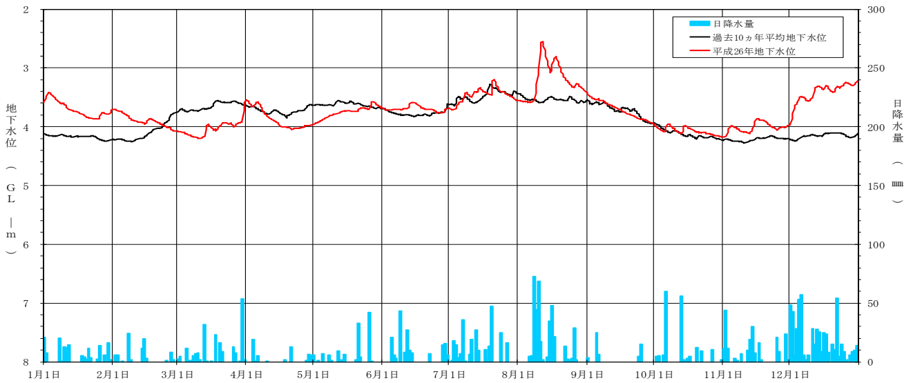
[ 平成 26 年地下水位変動グラフ 堂本 (浅) 観測井 (NO. 17) ]
