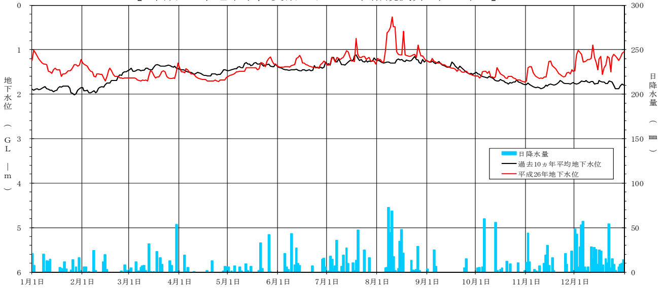
[平成26年地下水位変動グラフ 水落観測井 (NO.8) ]
