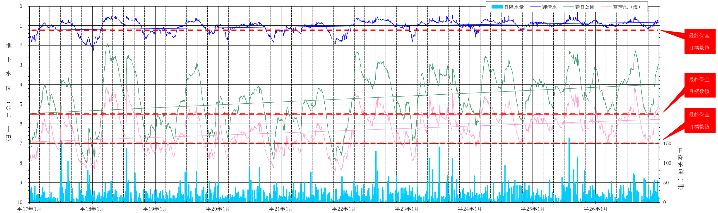
[ 3 観測井の地下水位変動グラフ (平成 17 年～26 年 10 年間) ]
