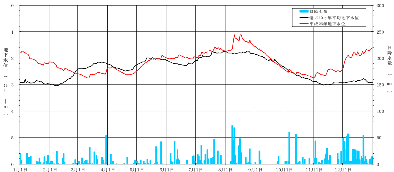
[ 平成 26 年地下水位変動グラフ 中挾観測井 (NO. 6) ]
