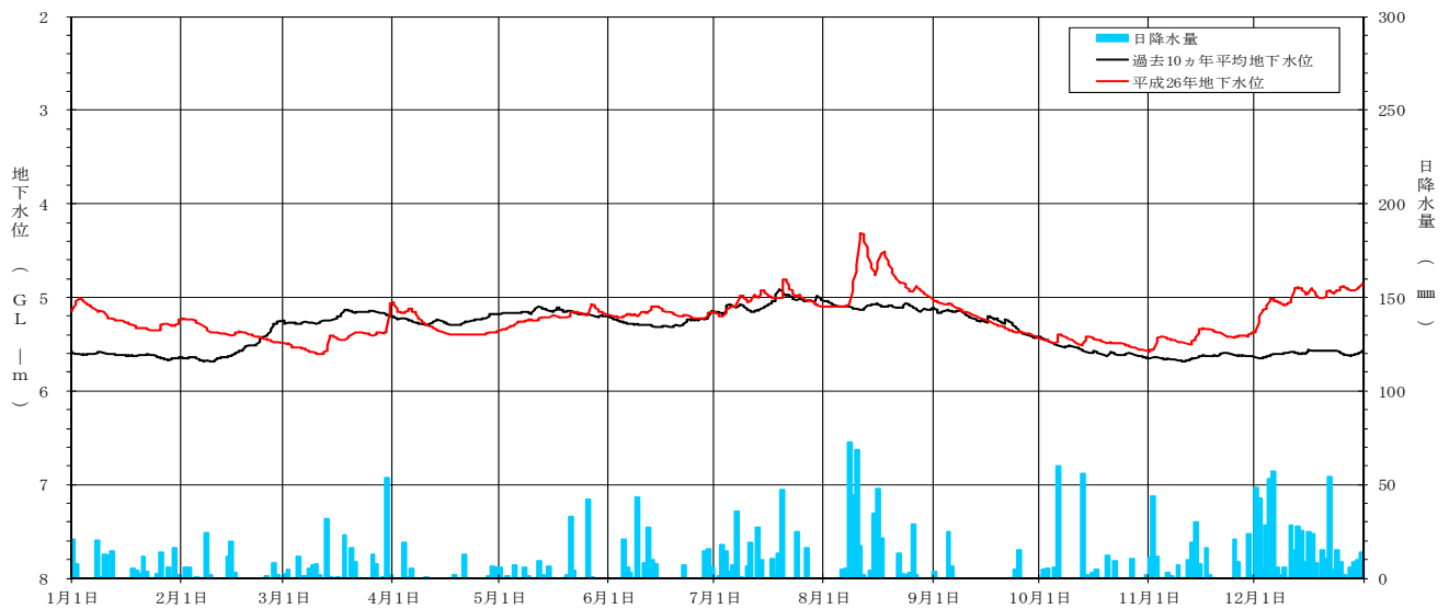
[ 平成 26 年地下水位変動グラフ 堂本 (深) 観測井 (NO. 18) ]
