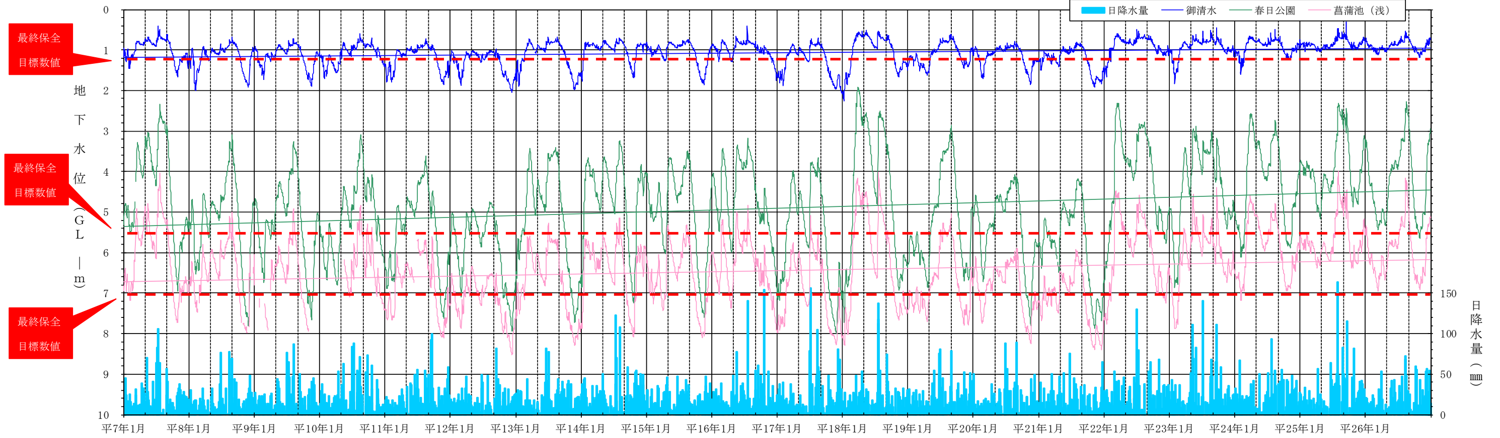
[ 3 観測井の地下水位変動グラフ (平成 7 年～26 年 20 年間) ]
