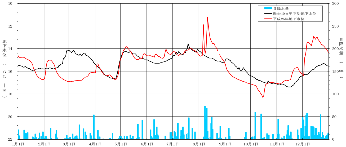
[ 平成 26 年地下水位変動グラフ 木本観測井（NO. 23） ]
