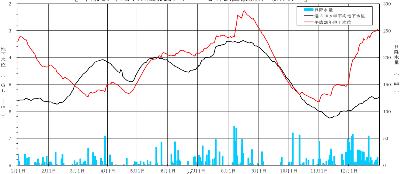
[ 平成 26 年地下水位変動グラフ 春日公園観測井 (NO. 3) ]
