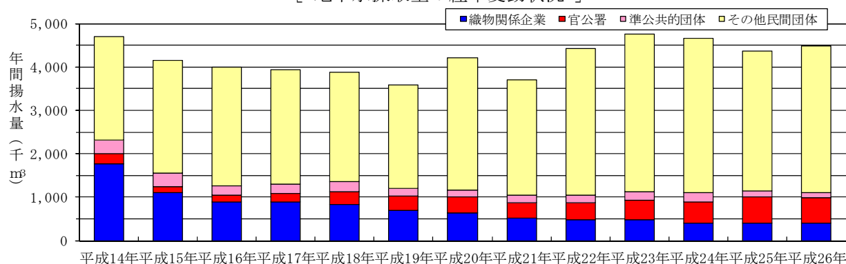
[ 地下水採取量の経年変動状況 ]
