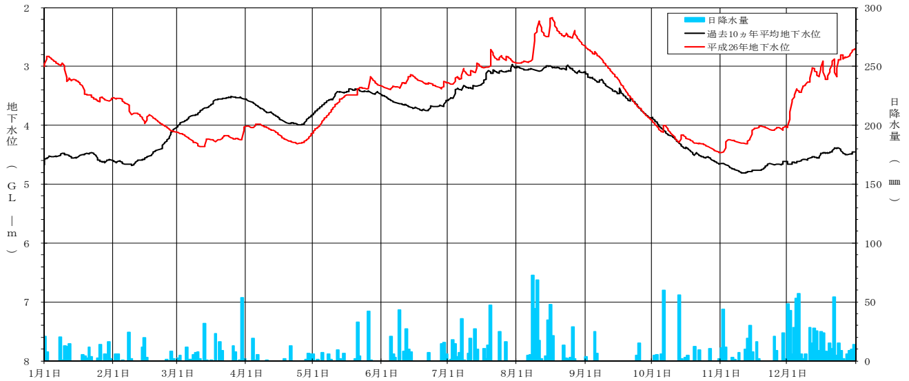
[ 平成 26 年地下水位変動グラフ 日吉 (浅) 観測井 (NO. 19) ]
