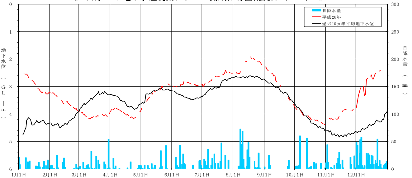
[ 平成 26 年地下水位変動グラフ 開成保育園観測井 (NO. 2) ]
