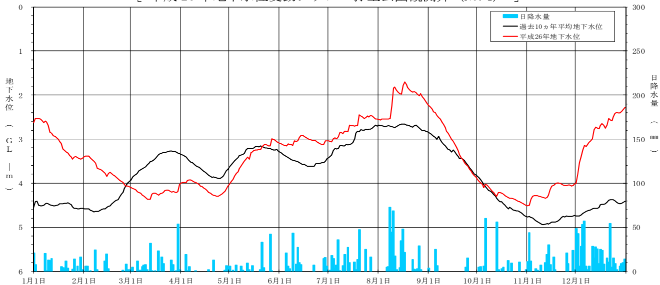
[ 平成 26 年地下水位変動グラフ 弥生公園観測井 (NO. 4) ]
