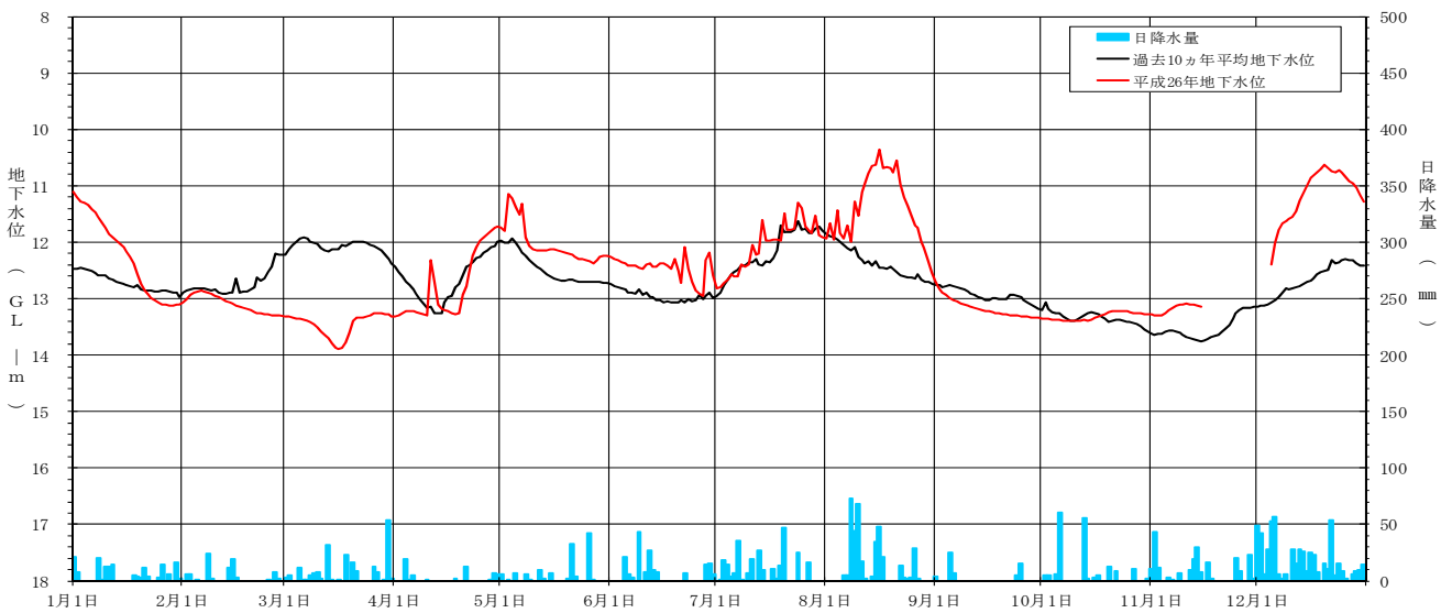
[ 平成 26 年地下水位変動グラフ 木本原上観測井 (NO. 26) ]
