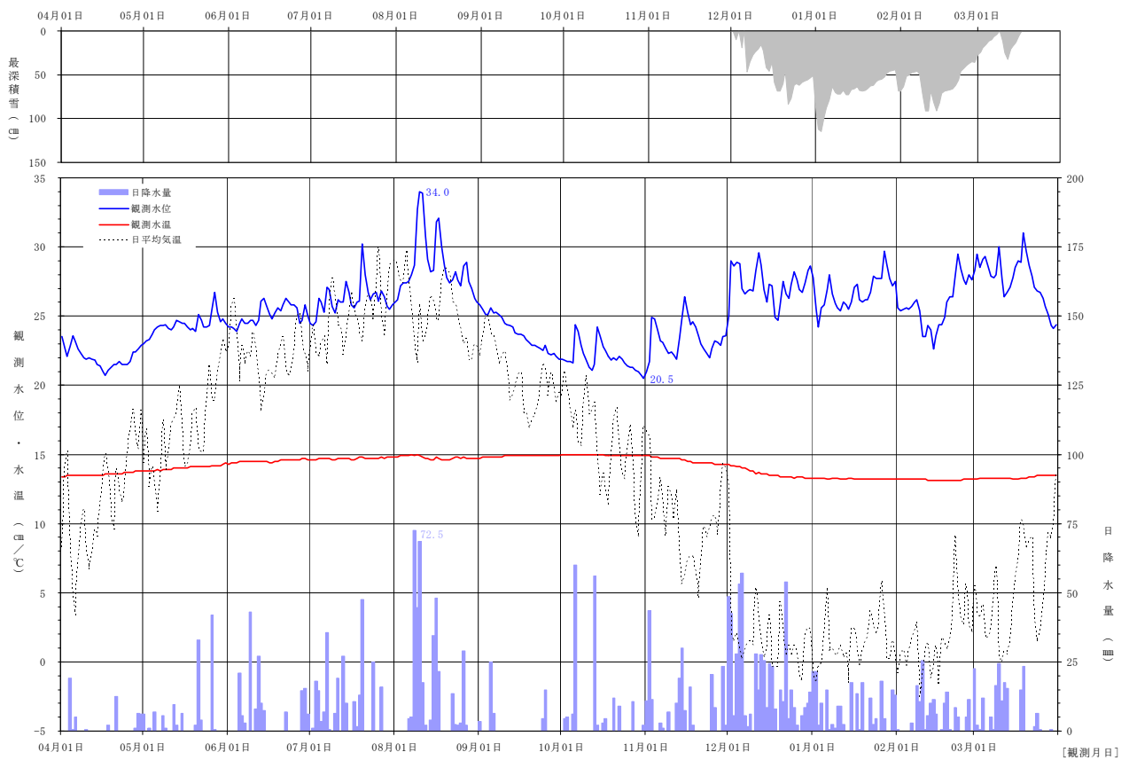
日水位・水温変動グラフ (中野清水)
