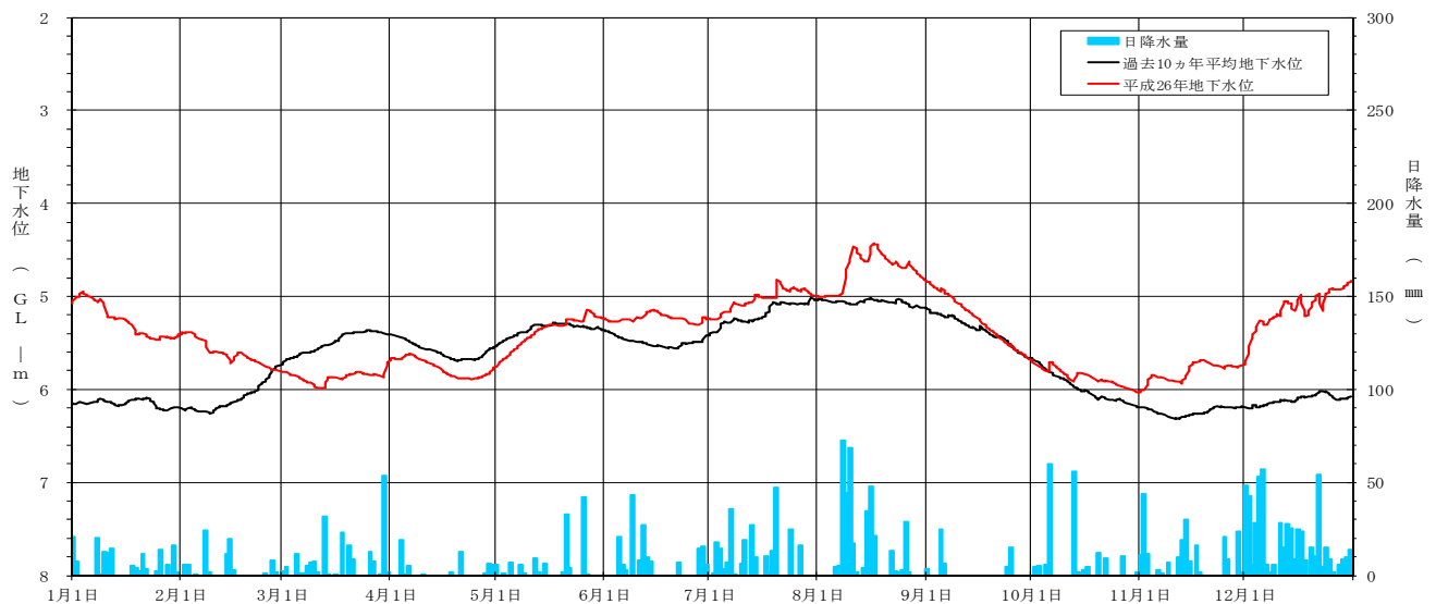
[ 平成 26 年地下水位変動グラフ 日吉 (深) 観測井 (NO. 20) ]
