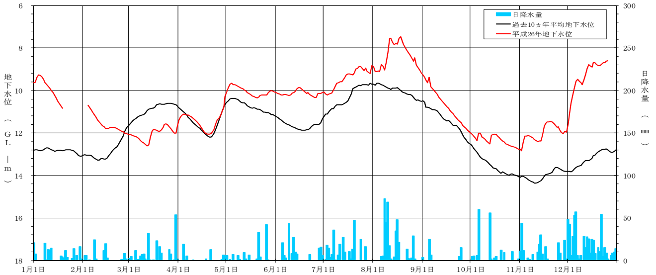
[ 平成 26 年地下水位変動グラフ 猪島観測井 (NO. 25) ]
