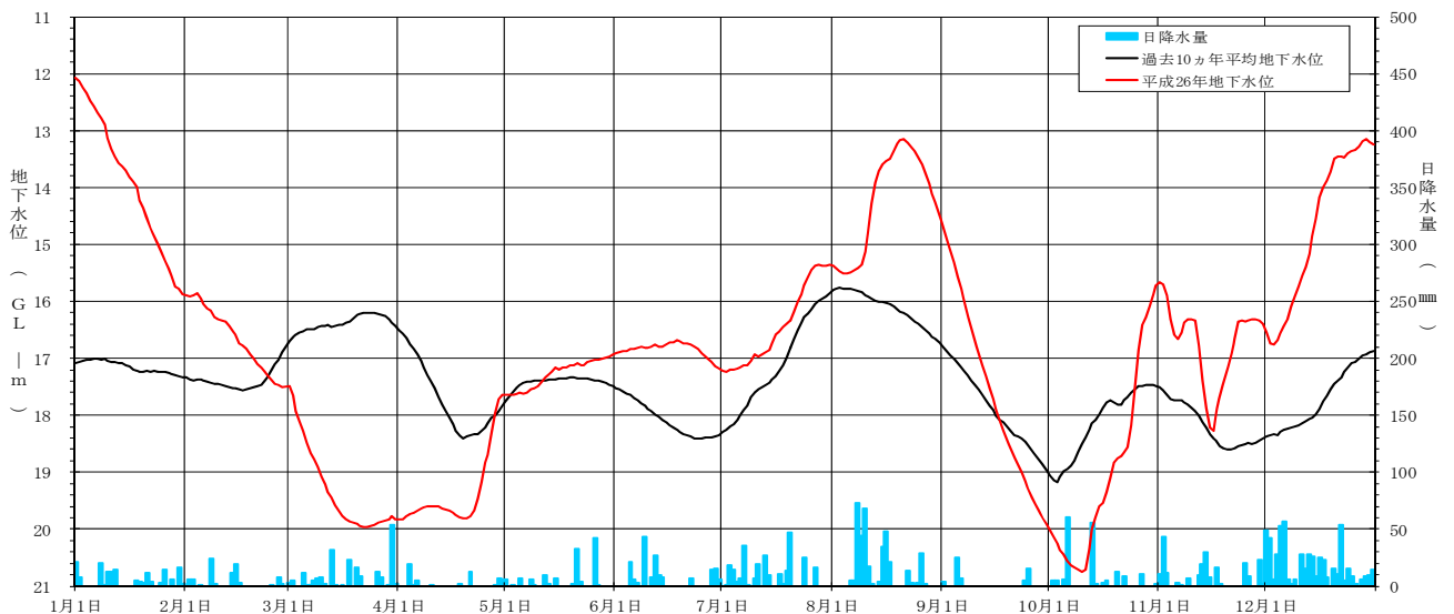
[ 平成 26 年地下水位変動グラフ 木本原中観測井 (NO. 27) ]
