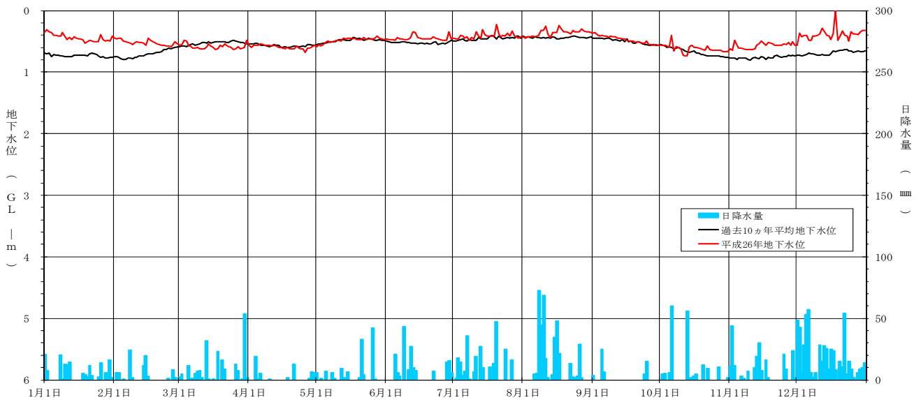
[ 平成 26 年地下水位変動グラフ 清瀧橋観測井 (NO. 14) ]
