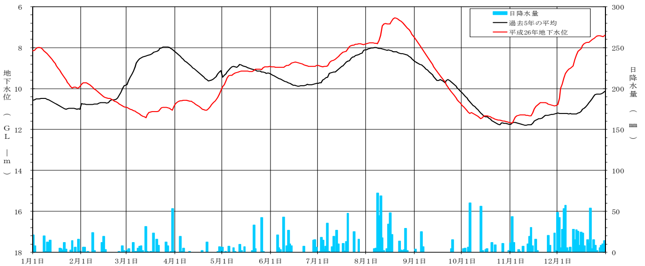
[ 平成 26 年地下水位変動グラフ 中据観測井 (NO. 29) ]
