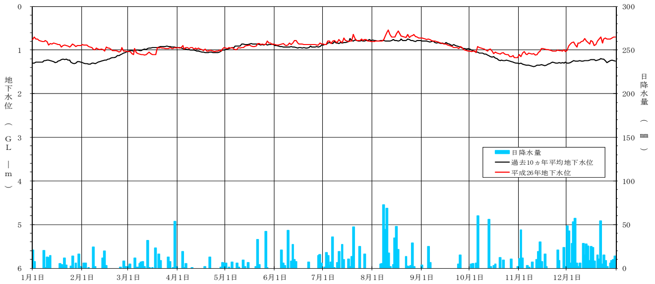
[平成26年地下水位変動グラフ 御清水観測井 (NO.7) ]
