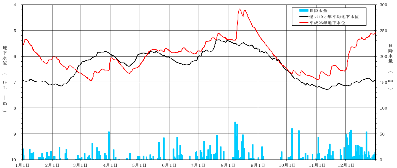
[ 平成 26 年地下水位変動グラフ 菖蒲池 (浅) 観測井 (NO. 21) ]
