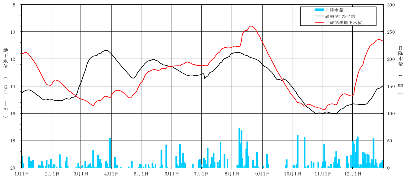
[ 平成 26 年地下水位変動グラフ 上据観測井 (NO. 30) ]
