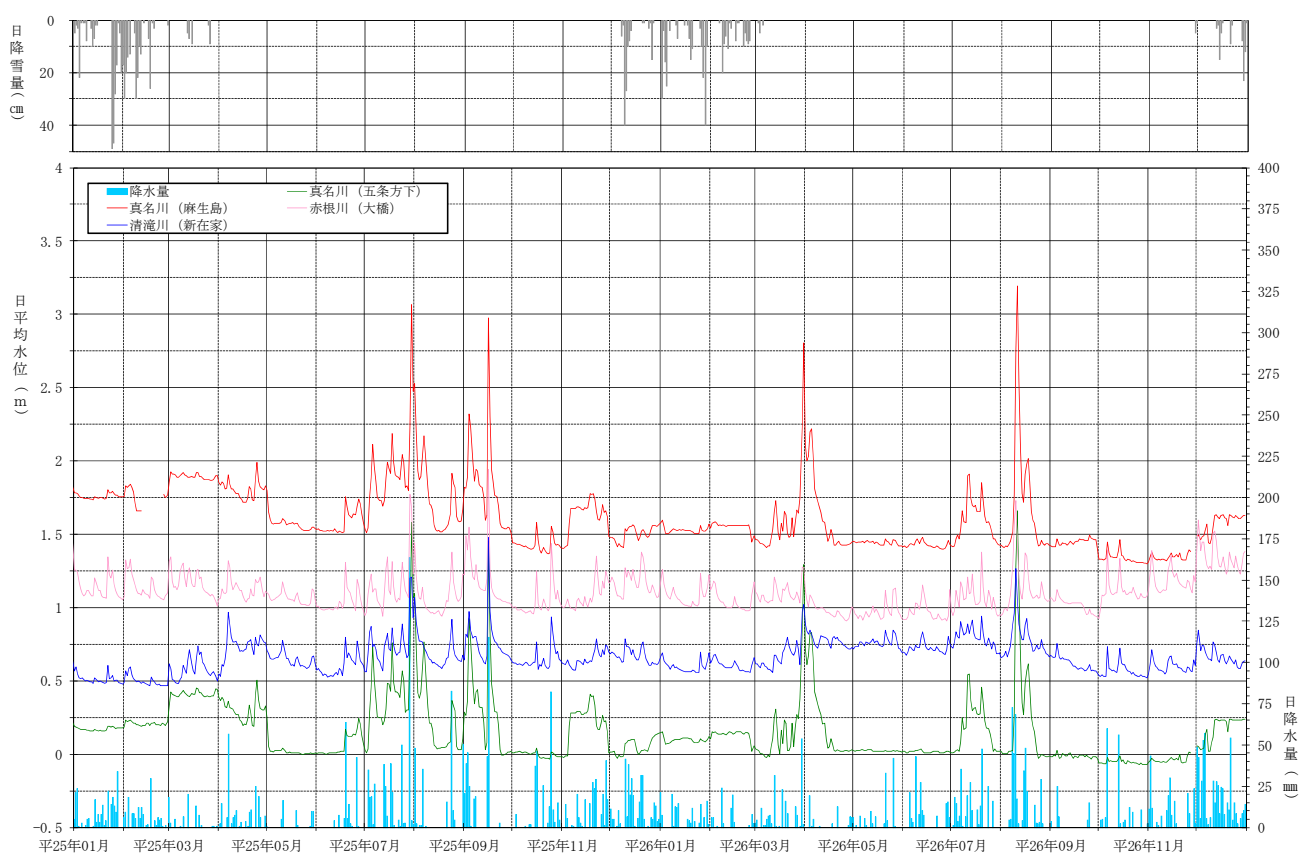
[ 河川水位の変動グラフ ] (平成 25 年 1 月～26 年 12 月)
