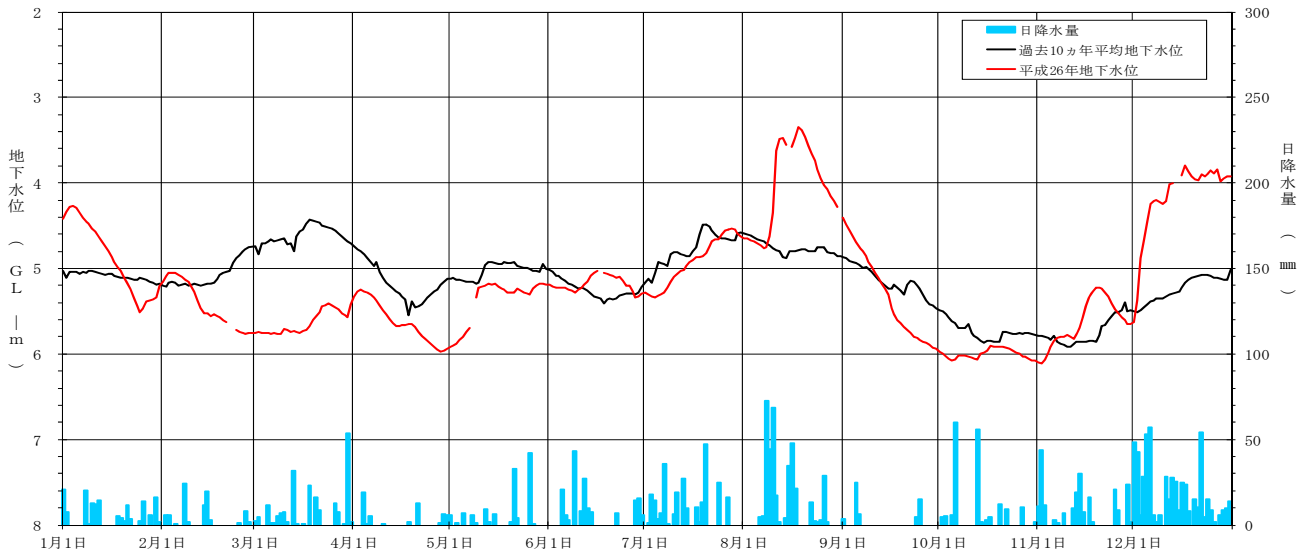
[ 平成 26 年地下水位変動グラフ 小山公民館観測井 (NO. 11) ]
