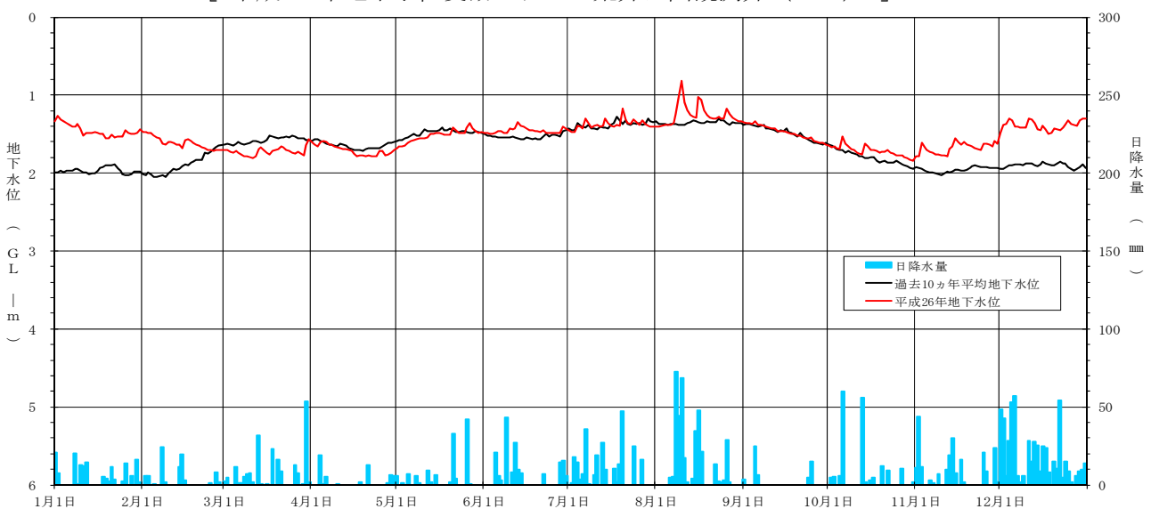
[平成26年地下水位変動グラフ 荒井公園観測井 (NO.9) ]
