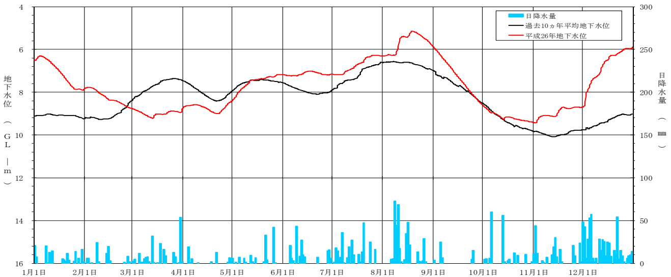
[ 平成 26 年地下水位変動グラフ 下据観測井 (NO. 15) ]
