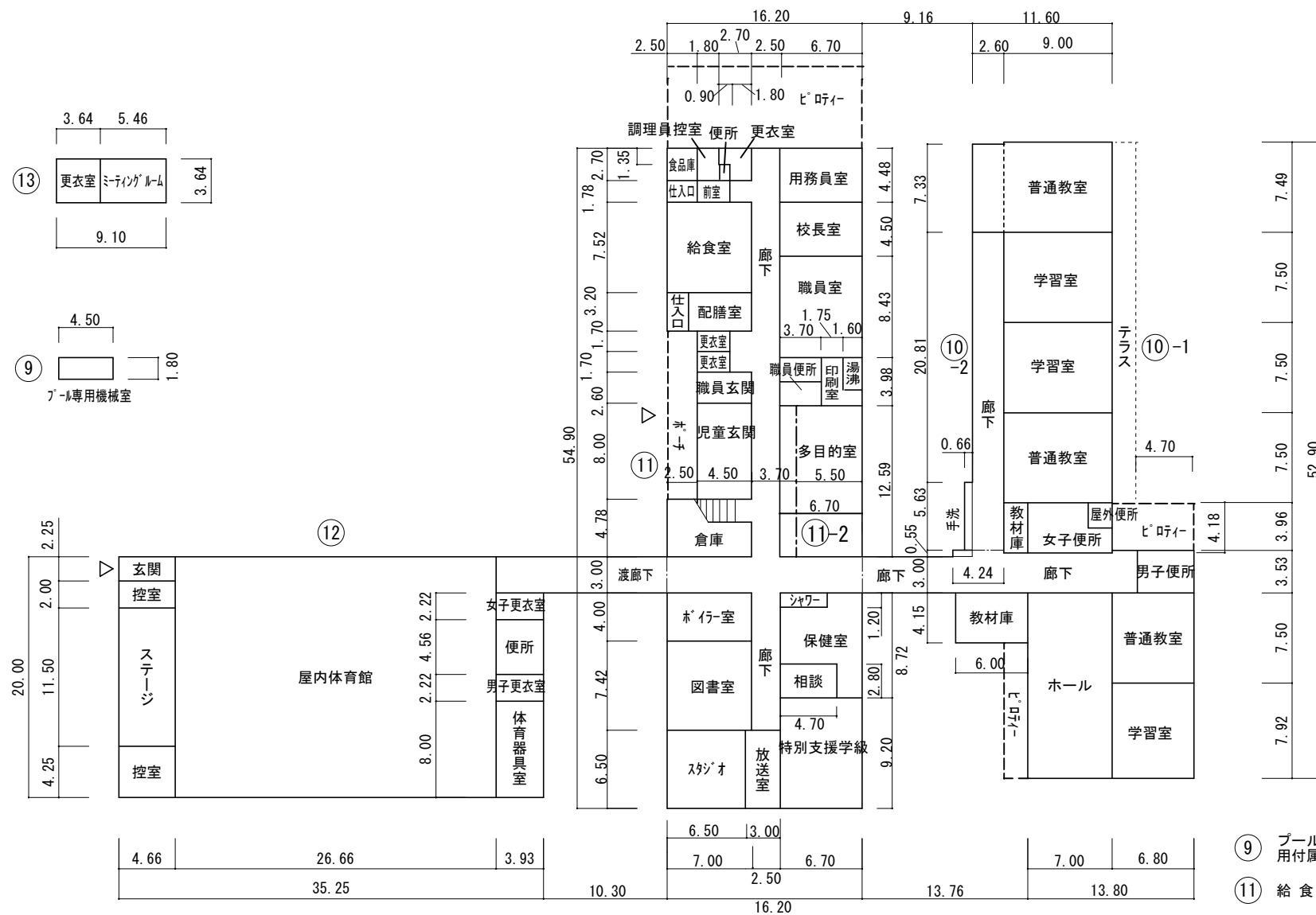
1階平面図 S=1:500
