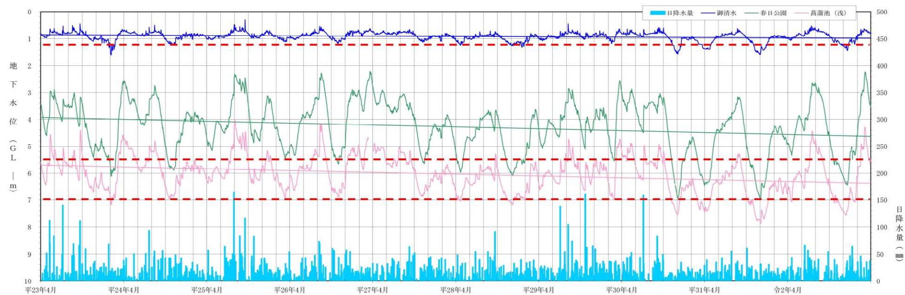
【3 観測井の地下水位変動グラフ（平成 23 年度～令和 2 年度 10 年間）】
