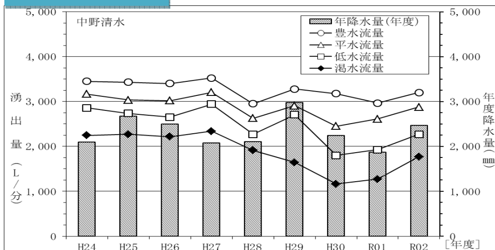
中野清水の流況の経年変化
