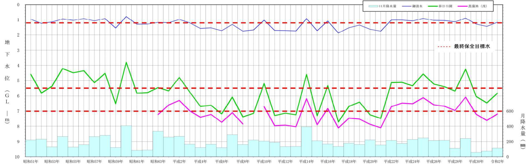
【基準観測井 11月平均地下水位の変動グラフ】
