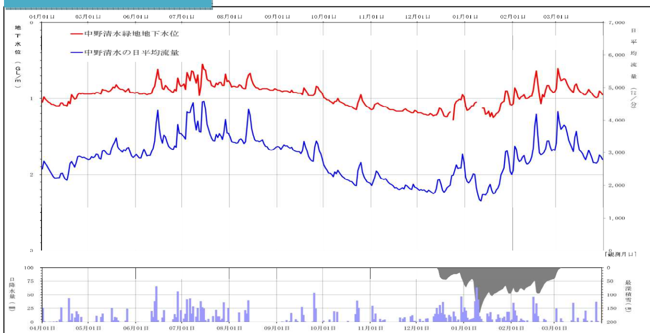
中野清水の地下水位と日平均流量
