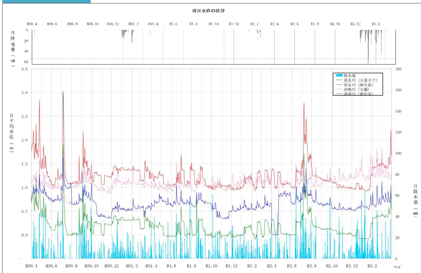
河川水位の変動グラフ
