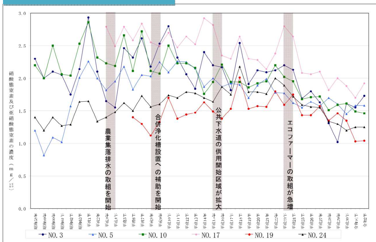
硝酸態窒素濃度及び亜硝酸態窒素濃度の経年変化
