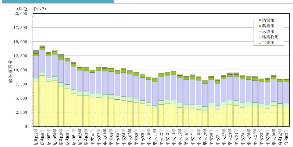
地下水の推計揚水量の経年変動グラフ
