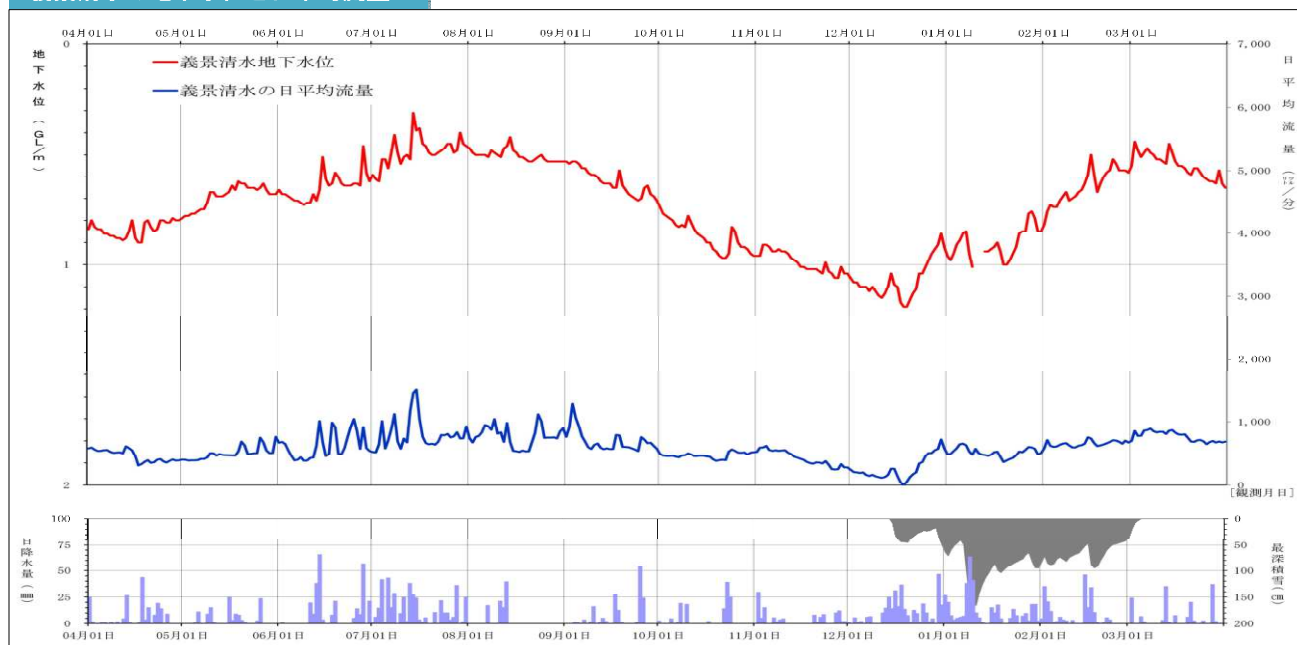
義景清水の地下水位と日平均流量
