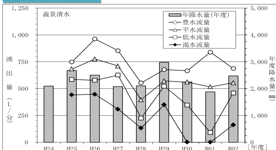
義景清水の流況の経年変化
