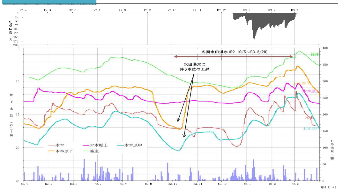
地下水位経年変動グラフ
