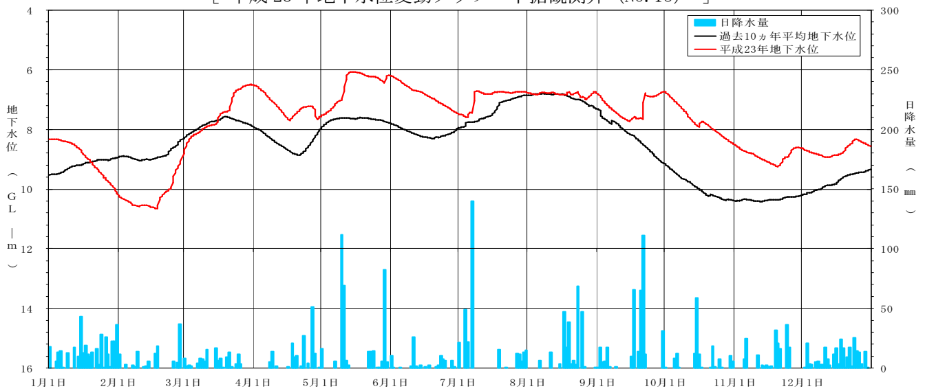
[ 平成 23 年地下水位変動グラフ 下据観測井 (NO. 15) ]
