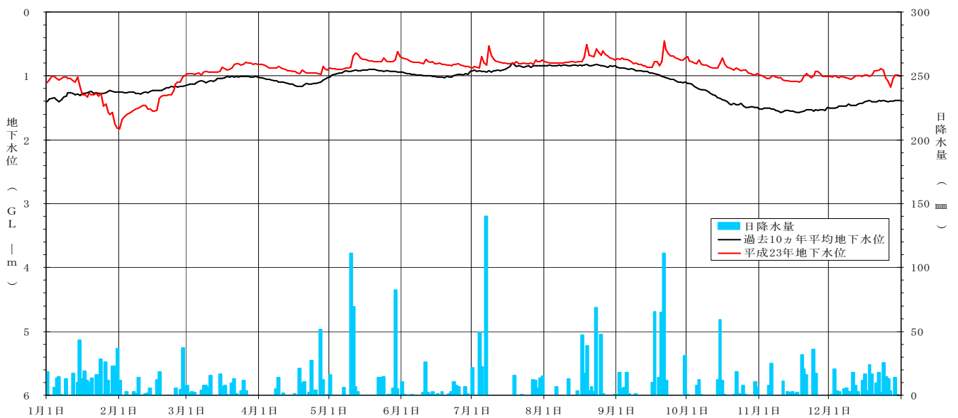
[ 平成 23 年地下水位変動グラフ 御清水観測井 (NO. 7) ]
