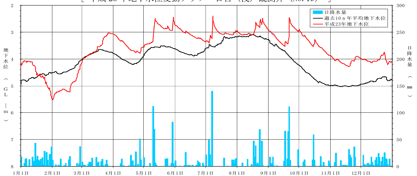
[ 平成 23 年地下水位変動グラフ 日吉（浅）観測井（NO.19） ]
