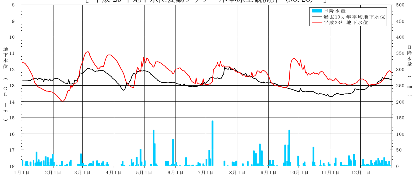
[ 平成 23 年地下水位変動グラフ 木本原上観測井 (NO. 26) ]
