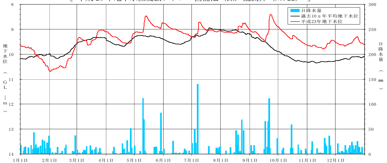
[ 平成 23 年地下水位変動グラフ 菖蒲池（深）観測井（NO. 22） ]
