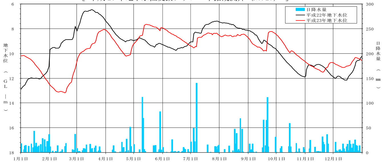
[ 平成 23 年地下水位変動グラフ 中据観測井 (NO. 29) ]
