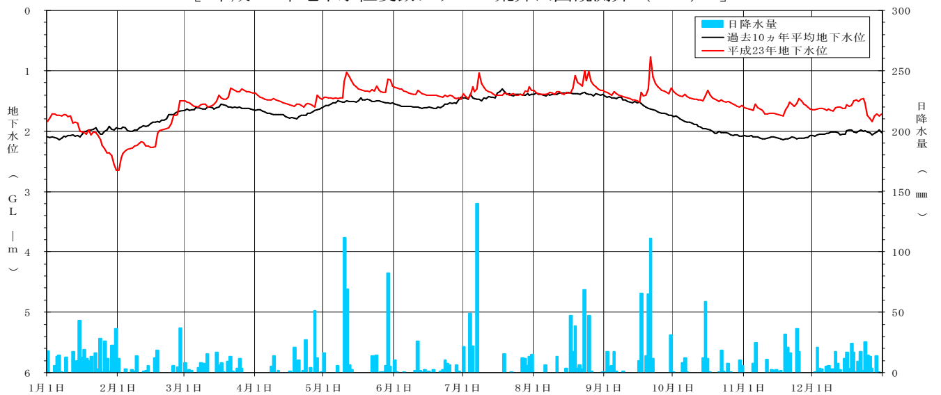
[ 平成 23 年地下水位変動グラフ 荒井公園観測井 (NO. 9) ]
