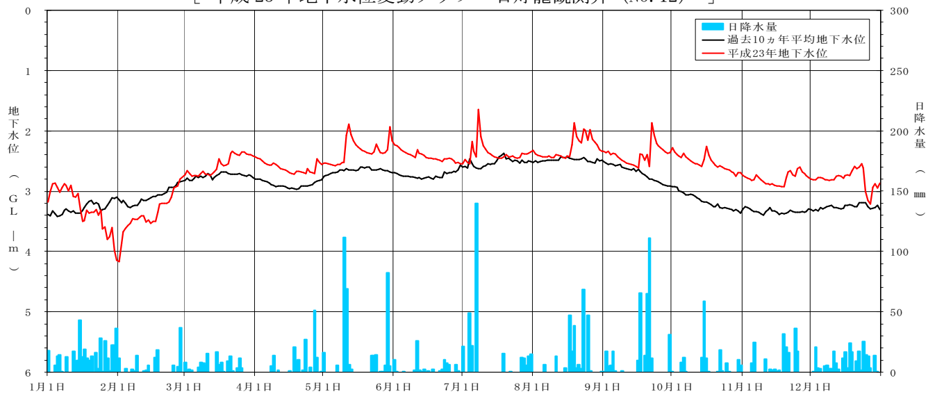
[ 平成 23 年地下水位変動グラフ 石灯籠観測井 (NO. 12) ]
