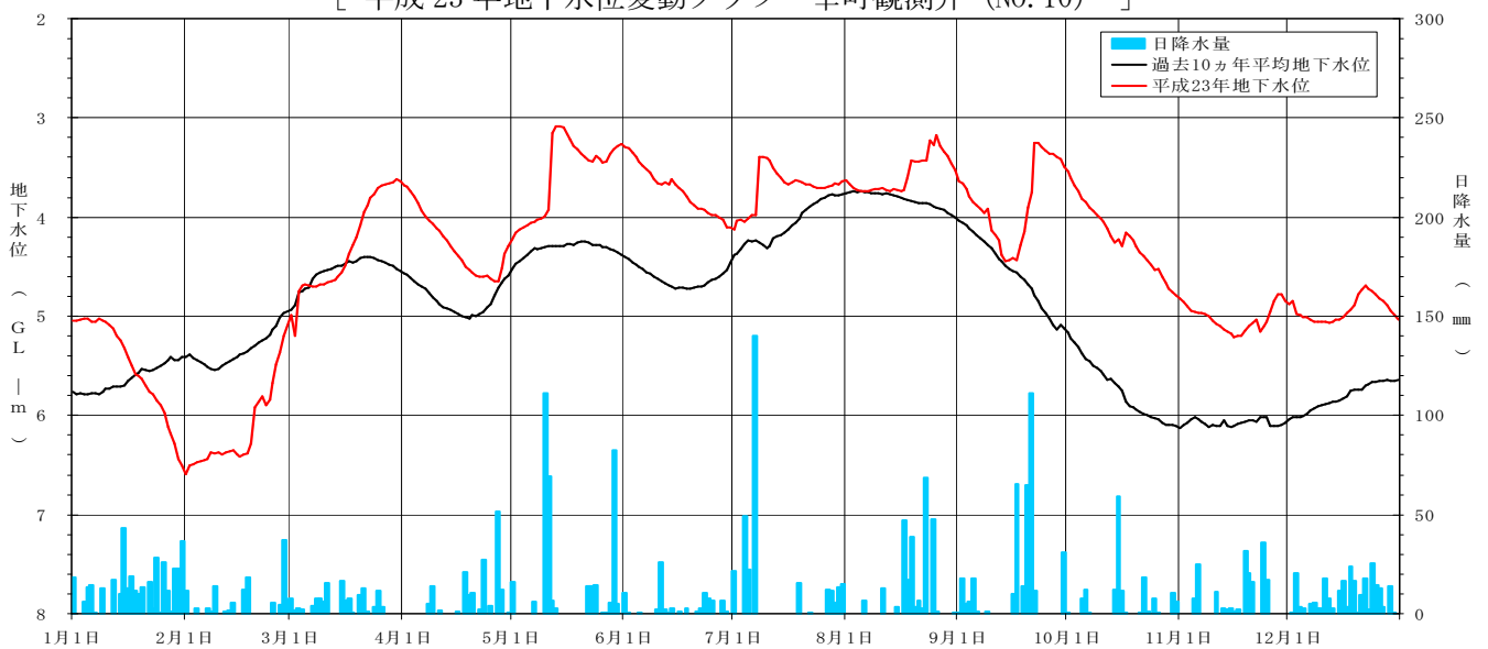
[ 平成 23 年地下水位変動グラフ 幸町観測井 (NO. 10) ]
