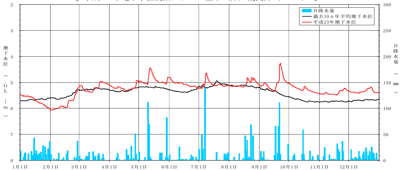
[ 平成 23 年地下水位変動グラフ 堂本（深）観測井（NO.18） ]
