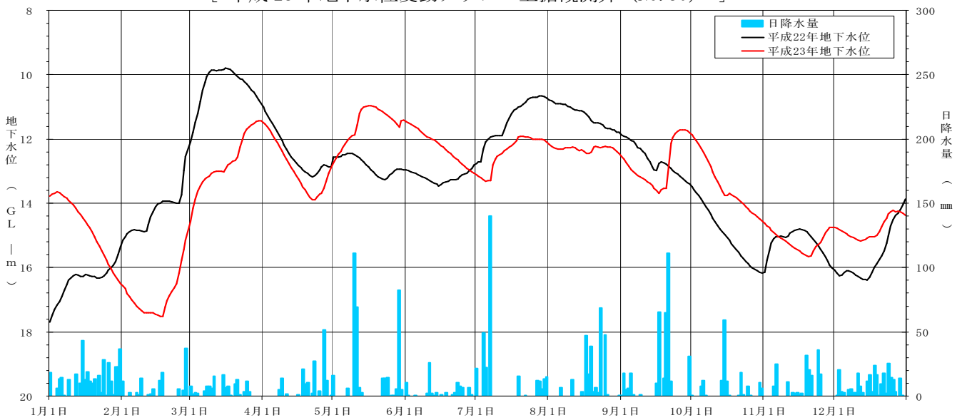
[ 平成 23 年地下水位変動グラフ 上据観測井 (NO. 30) ]
