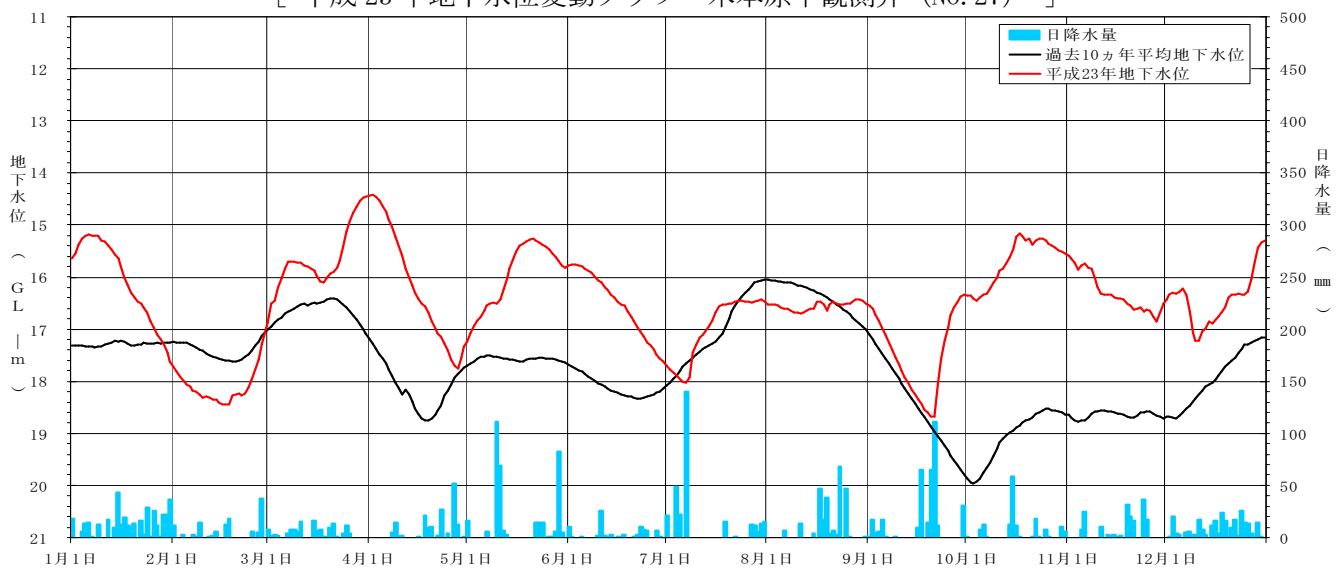
[ 平成 23 年地下水位変動グラフ 木本原中観測井 (NO. 27) ]
