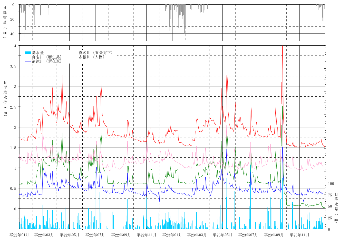
[ 河川水位の変動グラフ ] (平成 22 年 1 月～23 年 12 月)
