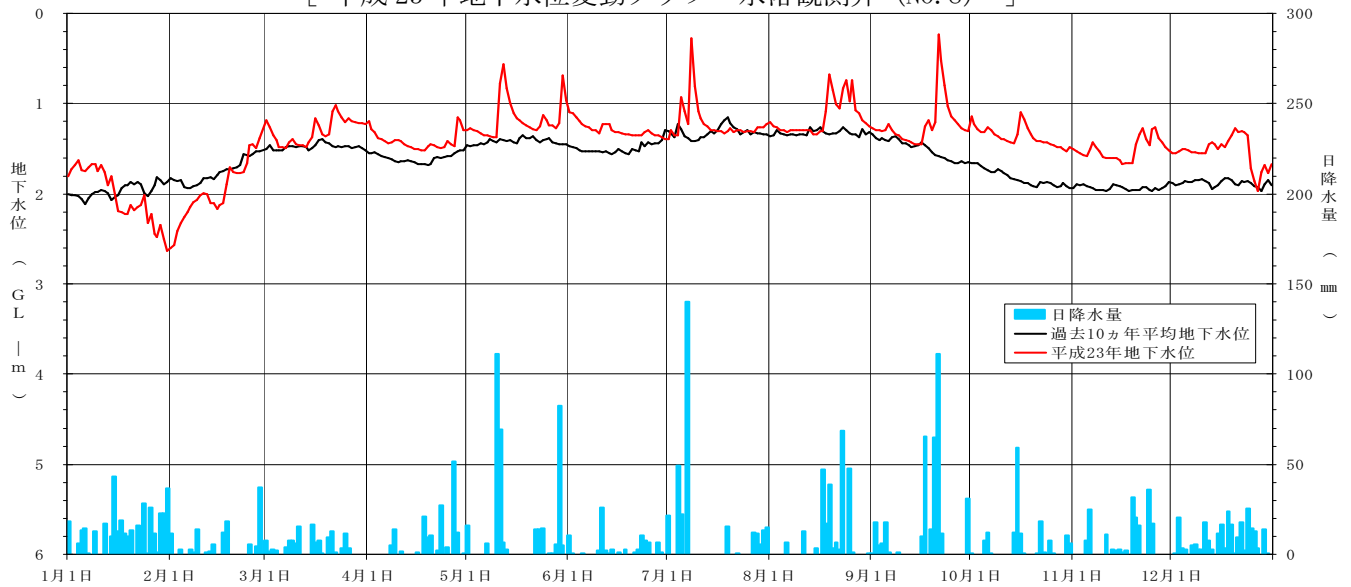
[ 平成 23 年地下水位変動グラフ 水落観測井 (NO. 8) ]
