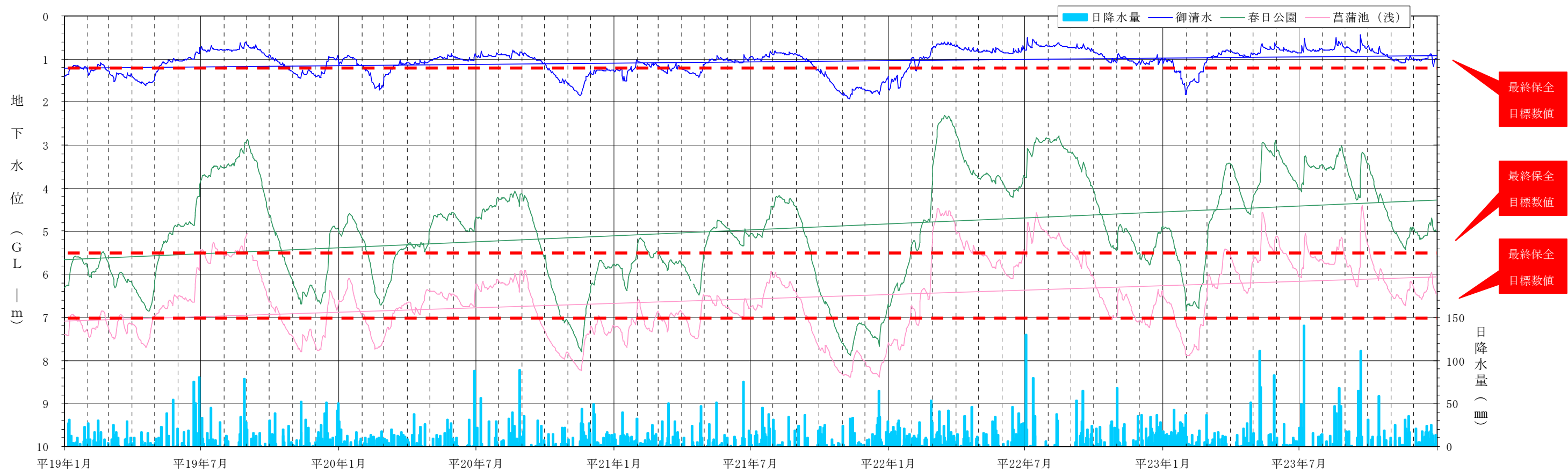
[ 3 観測井の地下水位変動グラフ（平成 19 年～23 年 5 年間） ]
