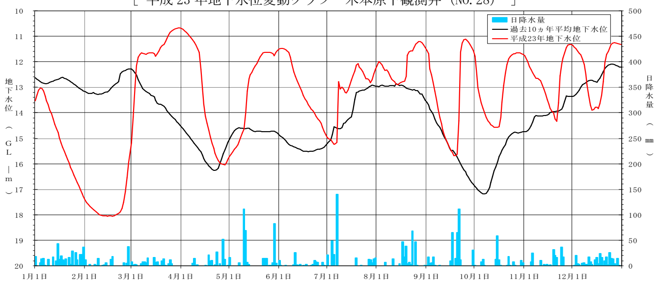
[ 平成 23 年地下水位変動グラフ 木本原下観測井 (NO. 28) ]
