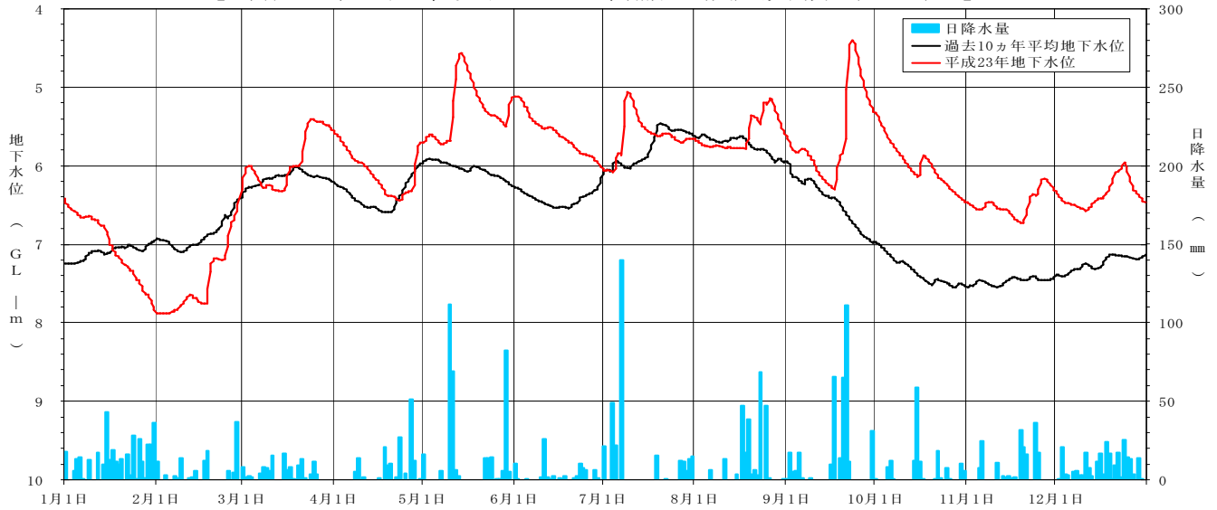
[ 平成 23 年地下水位変動グラフ 菖蒲池（浅）観測井（NO. 21） ]
