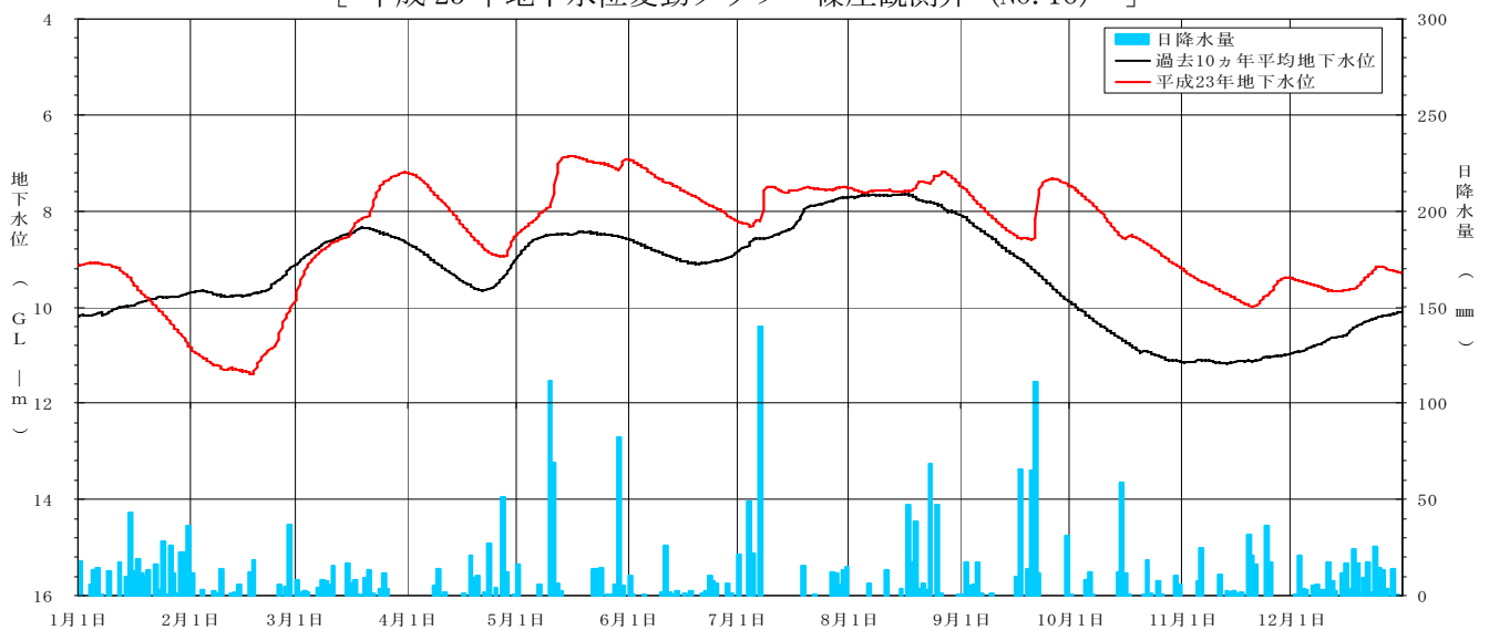
[ 平成 23 年地下水位変動グラフ 篠座観測井 (NO. 16) ]
