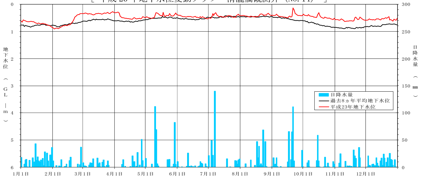
[ 平成 23 年地下水位変動グラフ 清瀧橋観測井 (NO. 14) ]
