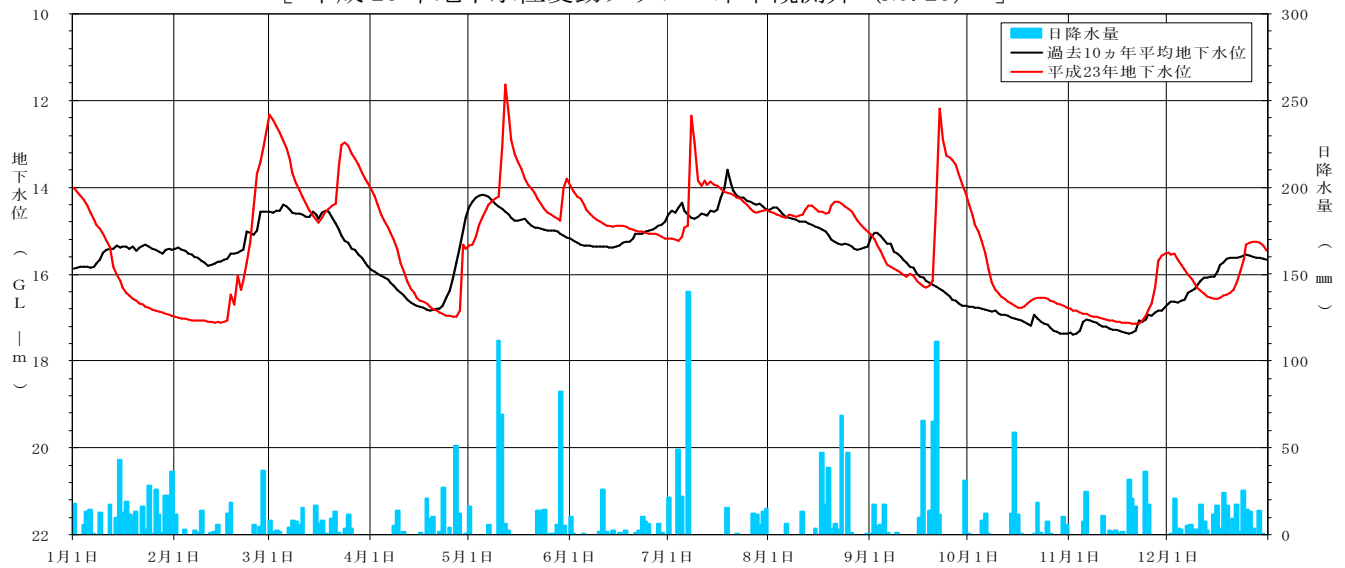
[ 平成 23 年地下水位変動グラフ 木本観測井 (NO. 23) ]
