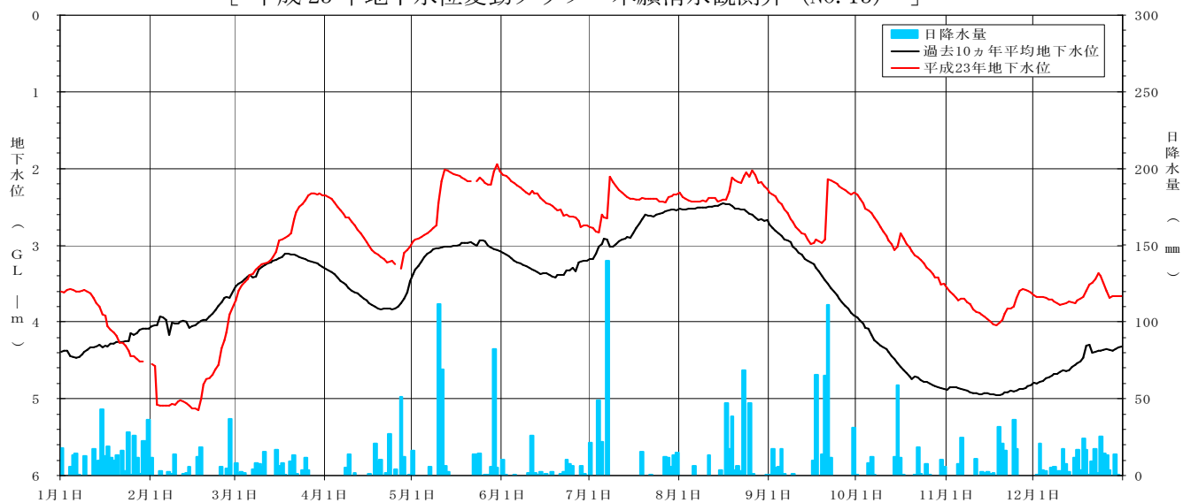
[ 平成 23 年地下水位変動グラフ 本願清水観測井 (NO. 13) ]
