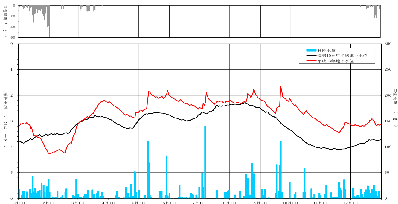
[ 平成23年地下水位変動グラフ 天神町観測井 (N0.1) ]
