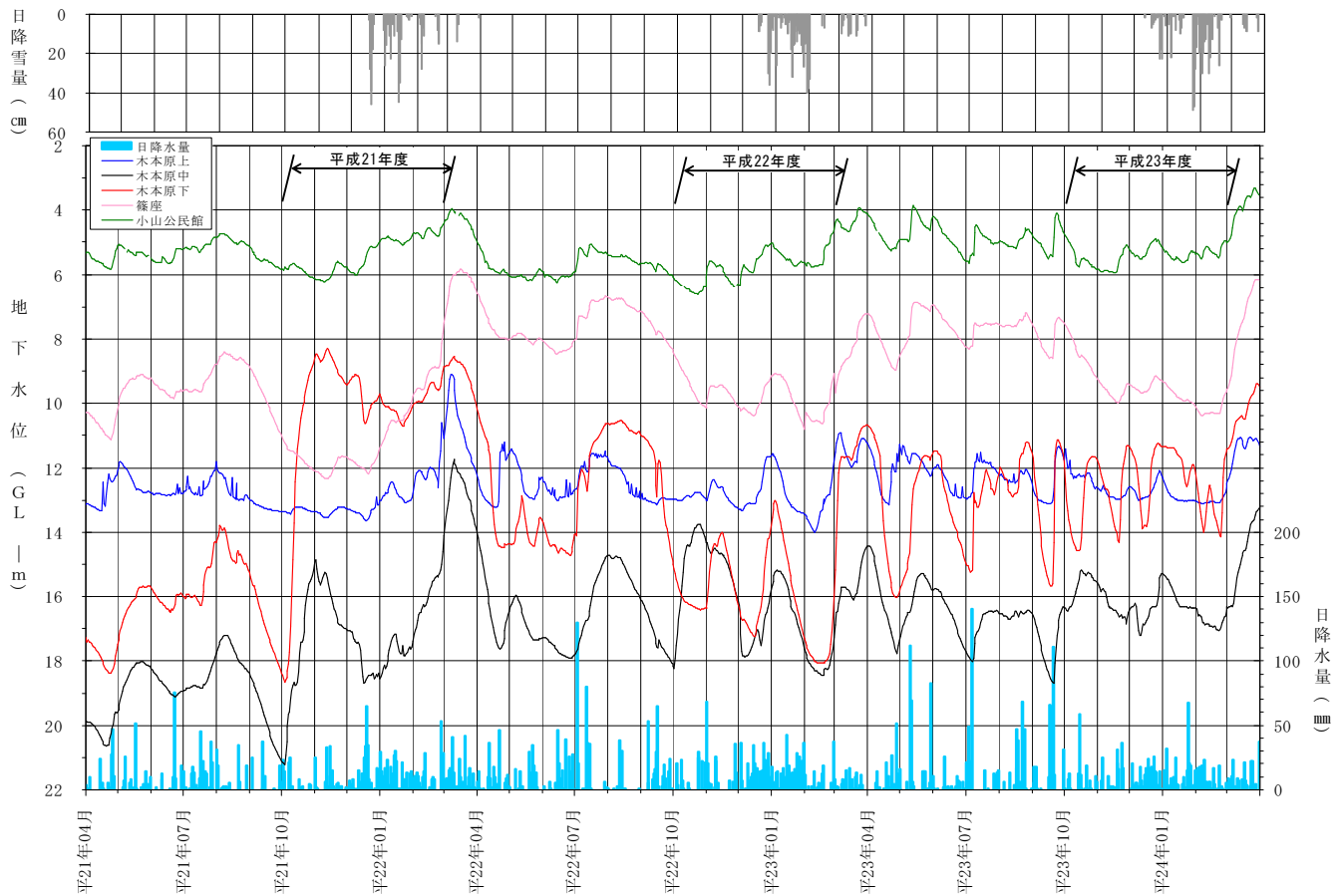
〔 地下水位経年変動グラフ（平成 21 年度～23 年度） 〕
