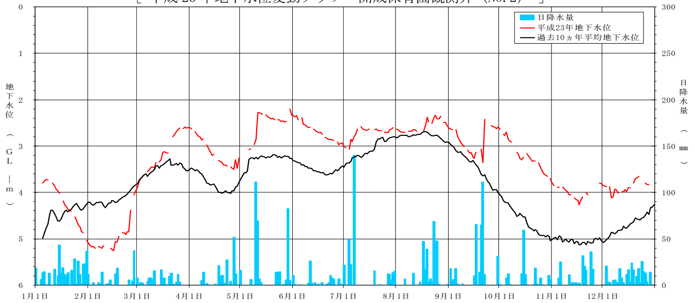
[ 平成 23 年地下水位変動グラフ 開成保育園観測井 (NO. 2) ]
