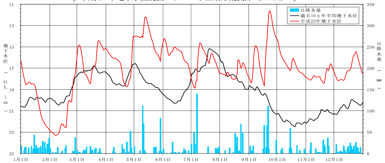
[ 平成 23 年地下水位変動グラフ 下五条方観測井 (NO. 24) ]
