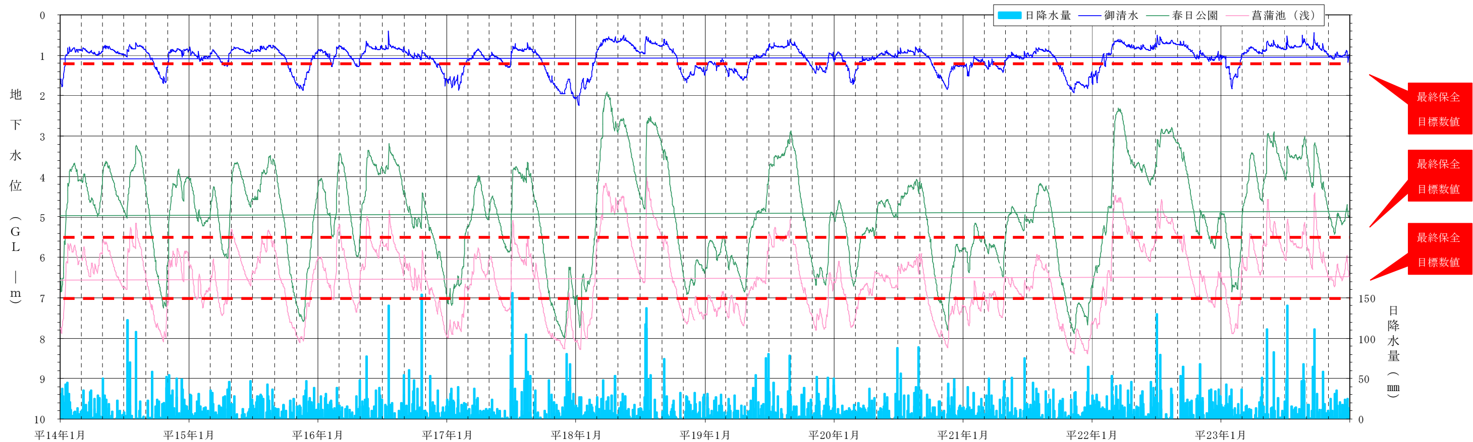
[ 3 観測井の地下水位変動グラフ（平成 14 年～23 年 10 年間） ]
