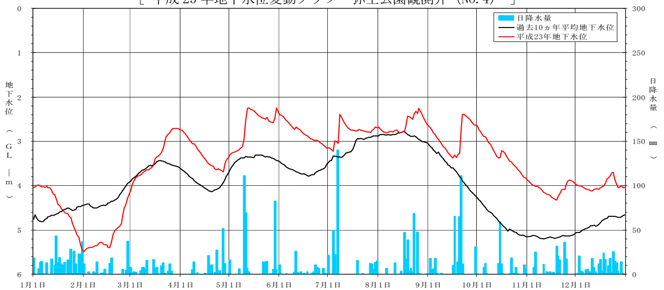
[ 平成 23 年地下水位変動グラフ 弥生公園観測井 (NO. 4) ]
