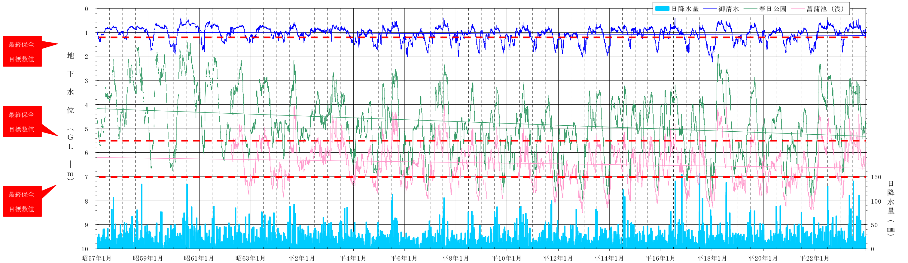
[ 3 観測井の地下水位変動グラフ（昭和 57 年～23 年 30 年間） ]
