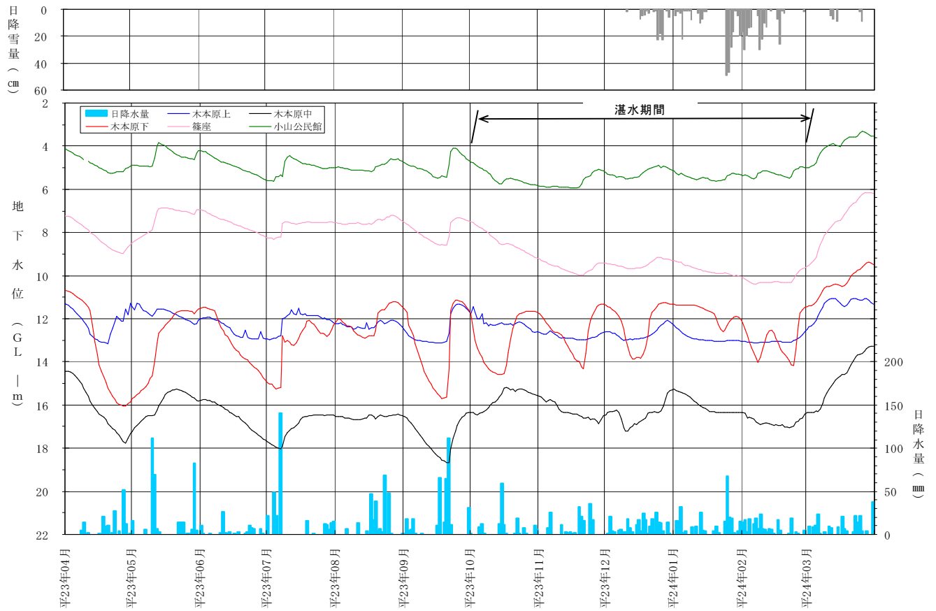
〔 地下水位年間変動グラフ（平成 23 年 4 月～24 年 3 月） 〕
