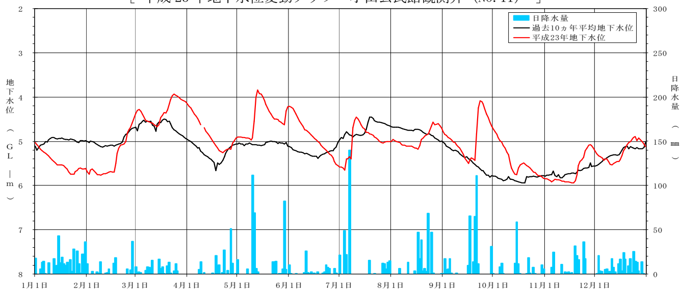
[ 平成 23 年地下水位変動グラフ 小山公民館観測井 (NO. 11) ]
