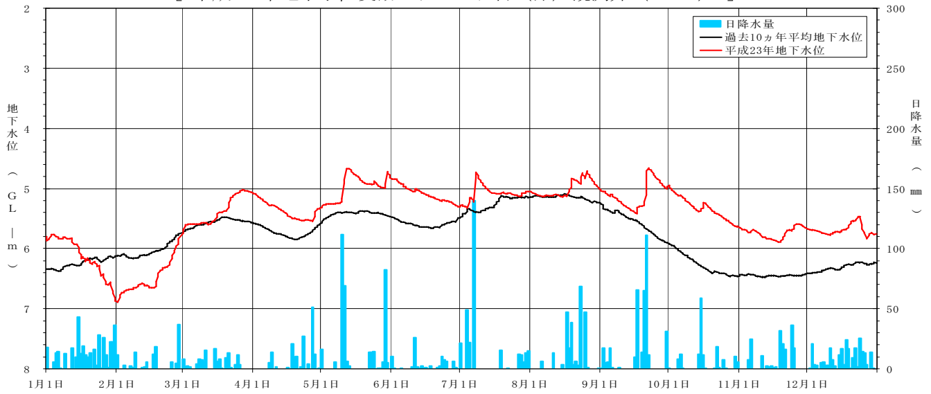
[ 平成 23 年地下水位変動グラフ 日吉（深）観測井（NO. 20） ]
