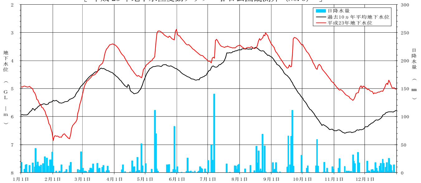
[ 平成 23 年地下水位変動グラフ 春日公園観測井 (NO. 3) ]
