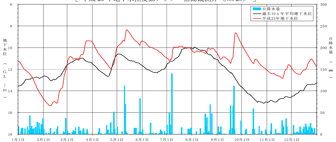
[ 平成 23 年地下水位変動グラフ 猪島観測井 (NO. 25) ]
