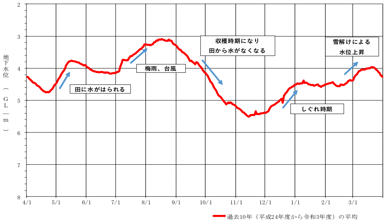
【春日公園観測井 過去10年の平均水位】
