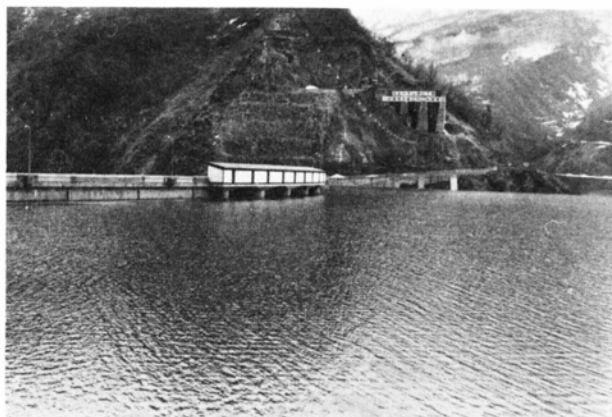
洪水時満水位（水深94 メートル ）に達した真名川ダム
