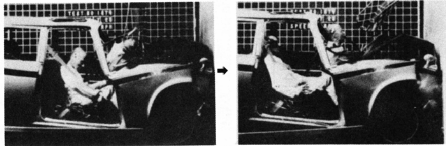
ダミーによる、シートベルト着用と非着用の比較。時速50kmでの衝突実験。
