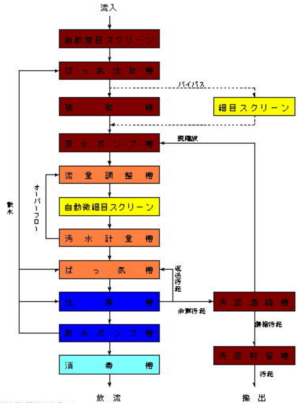
フローシート(例)
