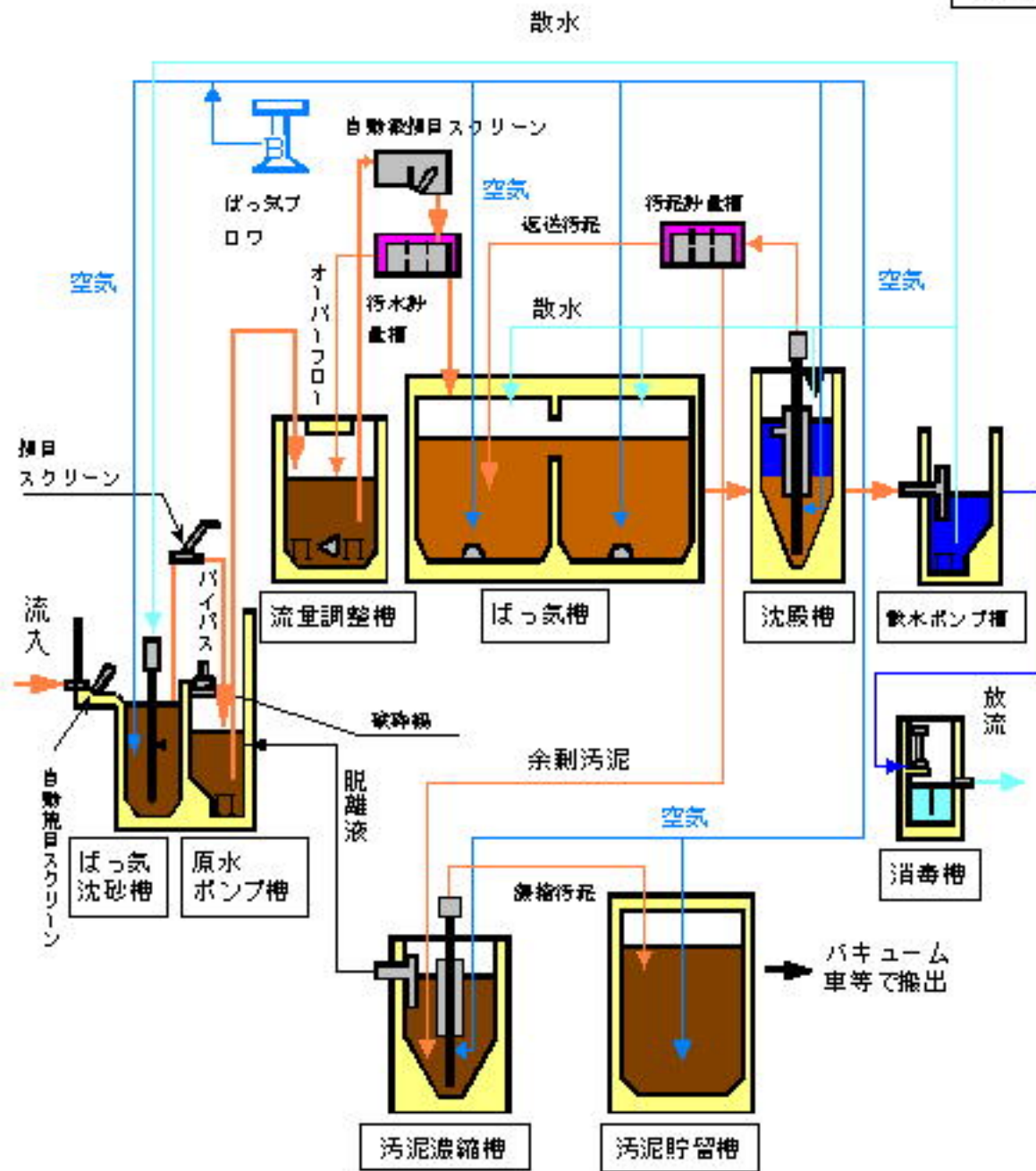
フローシート(例)
