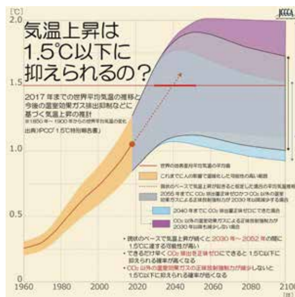
図表 3-2-1 1.5℃特別報告書
